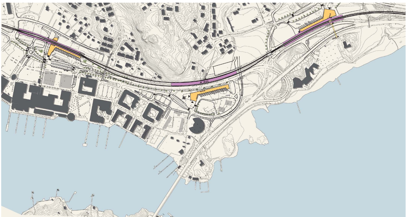
Situationsplan, Stenungsund
